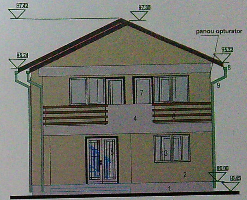
FATADA PRINCIPALA 1-sodu impermeabil; 2-tencuiala decorativa crem; 3-fereastră PVC nuanță lemn; 4-vopsea lavabilă albă; 5-usă metalică; 6-balustradă lemn; 7-usă PVC nuanță lemn; 8-igheab; 9-burlan
