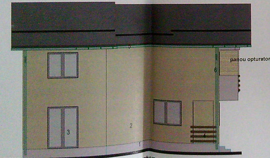
FATADA LATERALA STANGA 1-sodu impermeabil; 2-tencuiala decorativa crem; 3-fereastră PVC nuanță lemn; 4-balustradă lemn; 5-igheab; 6-burlan; 7-parazapezi
